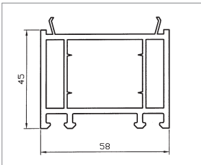
Blendrahmenverbreiterung, 45 mm
