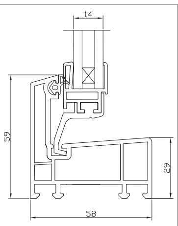
Isolierglas 14 mm
