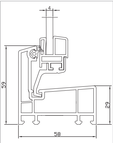
Dickglas 4 mm
